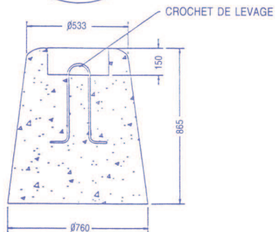
COUPE A-A
